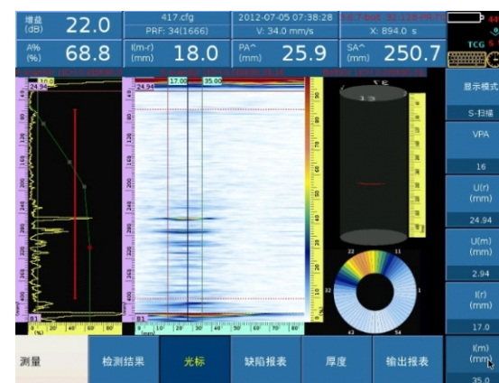
有裂纹螺栓检测图像
