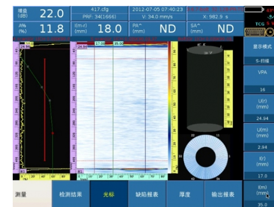
无裂纹螺栓检测图像
